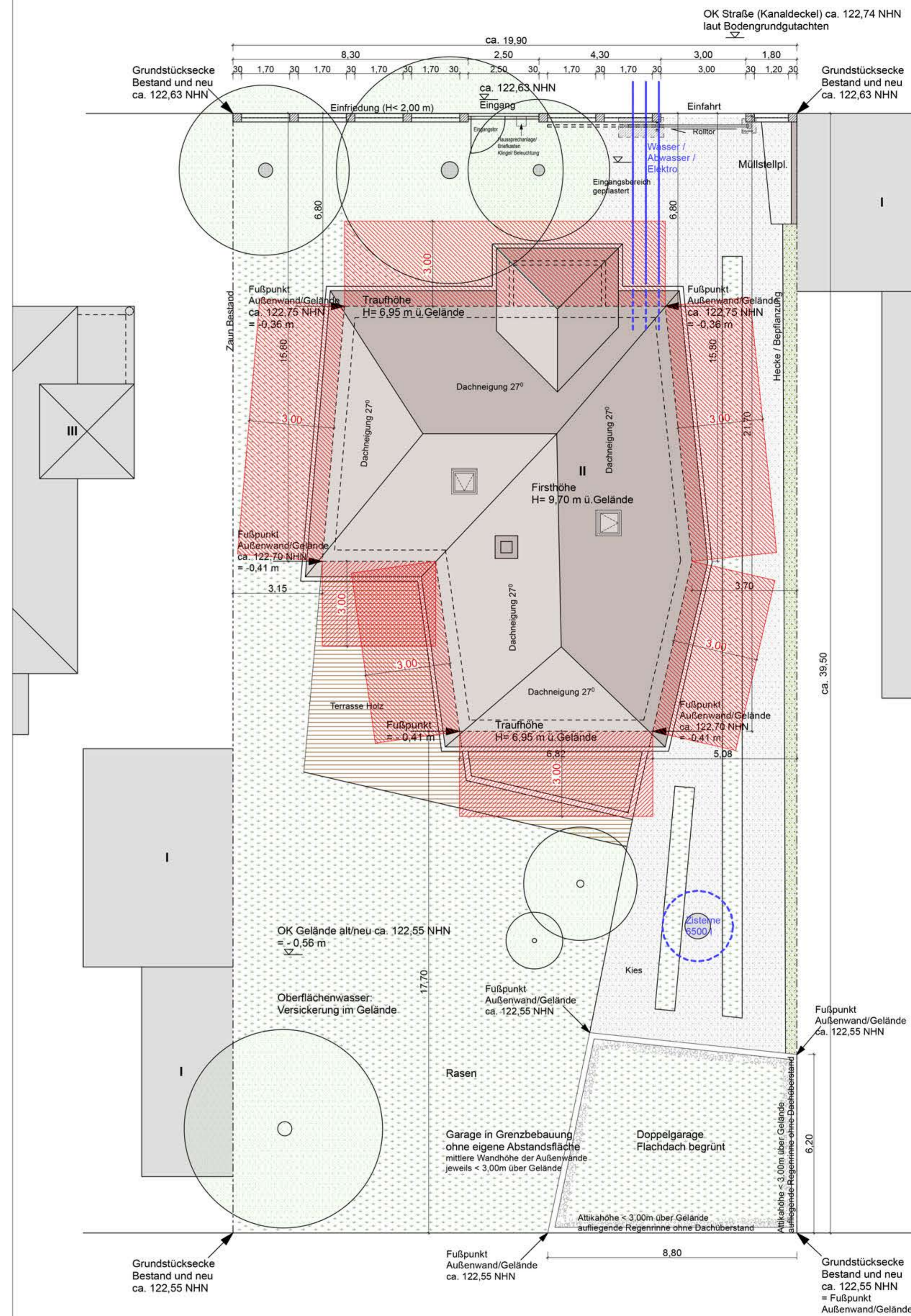
Lageplan M. 1.200
